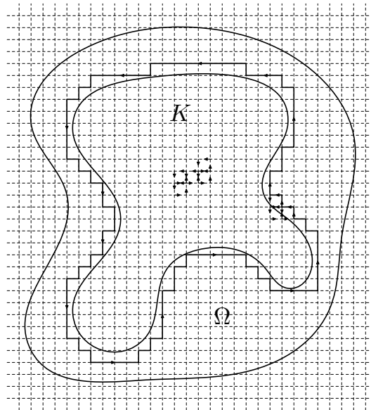
Figura 4.16: Ciclo que rodea un compacto
